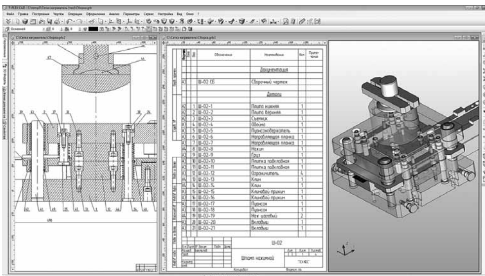
Рис. 2. 3D модель, спецификация и чертеж в одном документе
